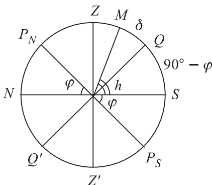
Рис. 3.4. К задаче о высоте светила в кульминации
