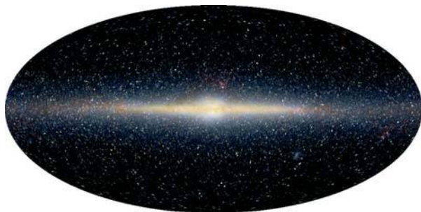
16. Развернутое изображение Млечного пути – звездного диска нашей Галактики. Космическая обсерватория КОБЕ (NASA)
