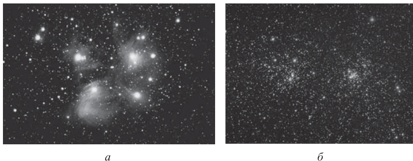
Рис. 28.2. Рассеянное скопление Плеяды в созвездии Тельца (а), рассеянные скопления \chi и h Персея (б)
