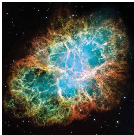
12. Крабовидная туманность – остаток сверхновой звезды, взрыв которой наблюдался в 1054 г. Расстояние до нее – 6,5 тыс. св. лет. Волокна туманности представляют собой нагретый газ. Природа голубоватого свечения внутри туманности иная, чем у газа: она связана с движением высокоэнергетичных электронов в слабом магнитном поле туманности. Космический телескоп “Хаббл” (NASA, группа HERITAGE)
