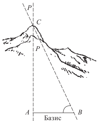
Рис. 8.5. Принцип определения расстояния по параллактическому смещению. Угол p — параллакс
