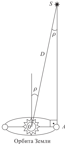
Рис. 22.1. Параллакс звезды
