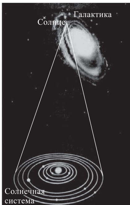
Рис. 1.3. Расположение Солнечной системы в Галактике
